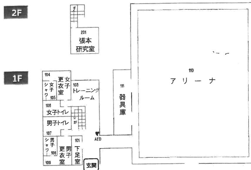
(F) 体育館平面図 (首里当蔵キャンパス)
