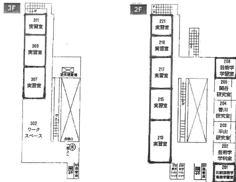
(E) 美術棟平面図 (首里当蔵キャンパス)
