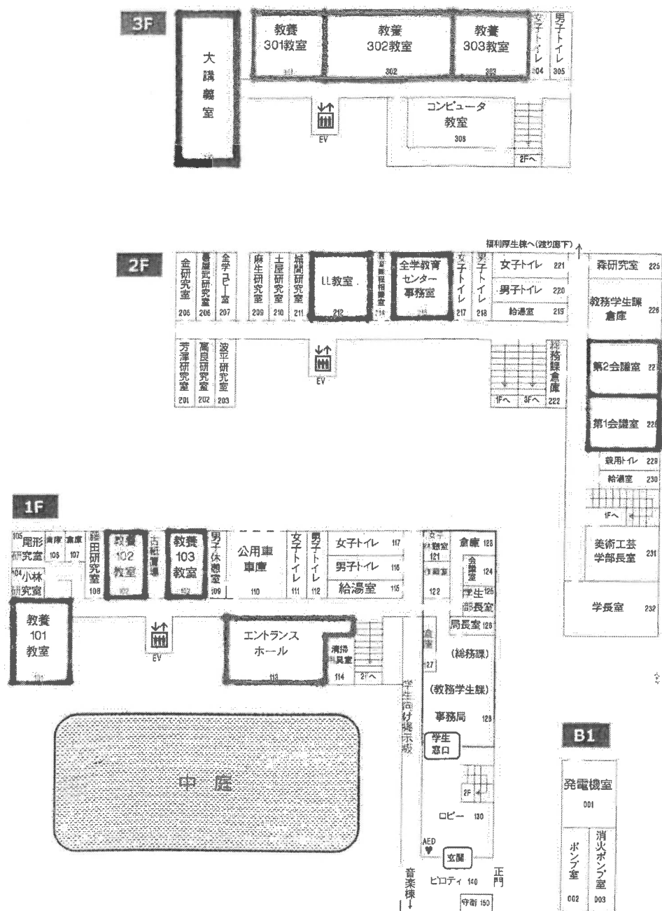
(A) 管理棟・一般教育棟平面図（首里当蔵キャンパス）
