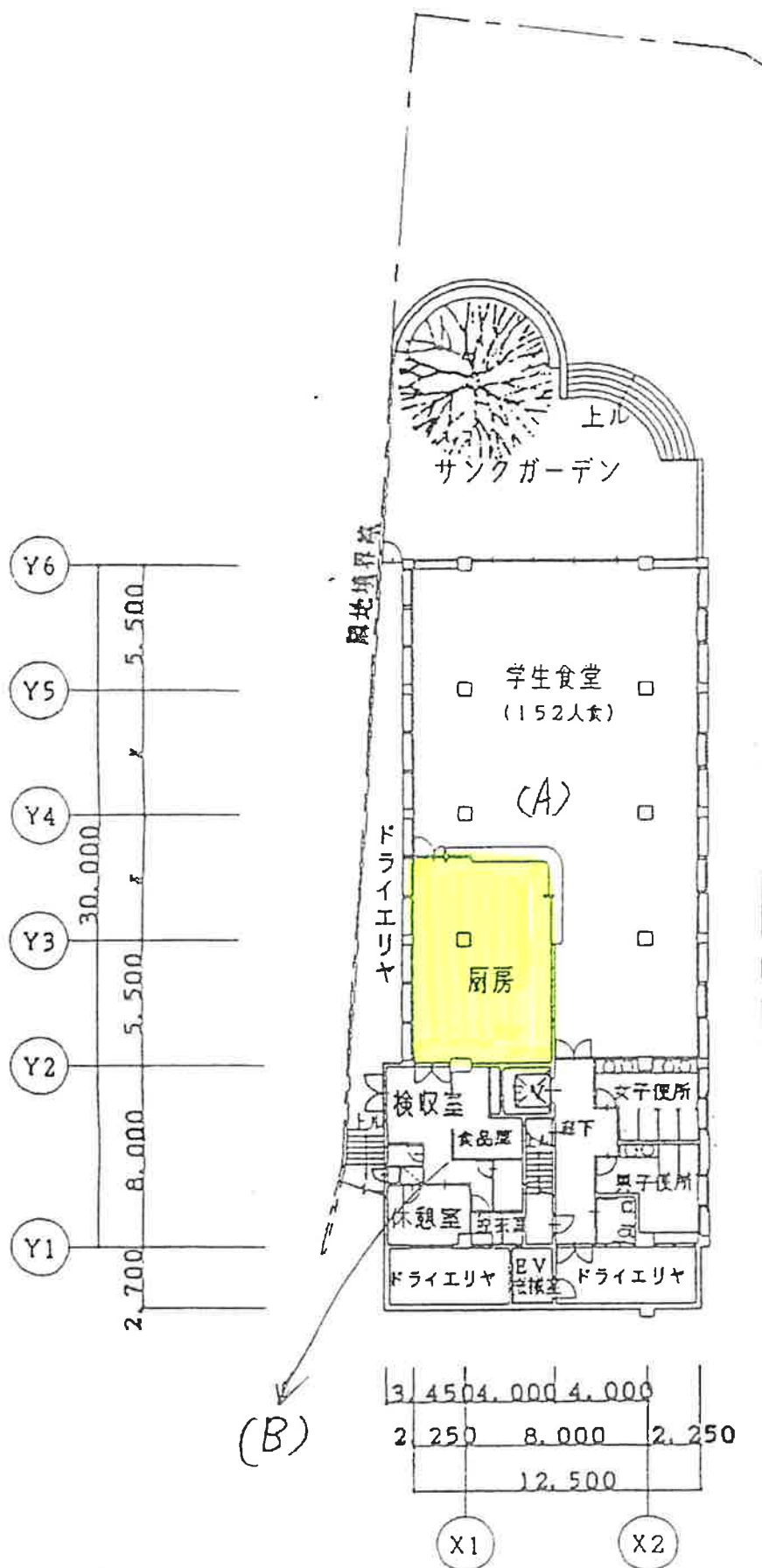
地下階平面図 S=1/500
